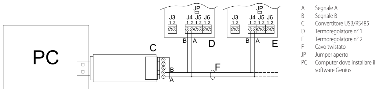
Figura 6.1 Schema di collegamento rete Modbus
